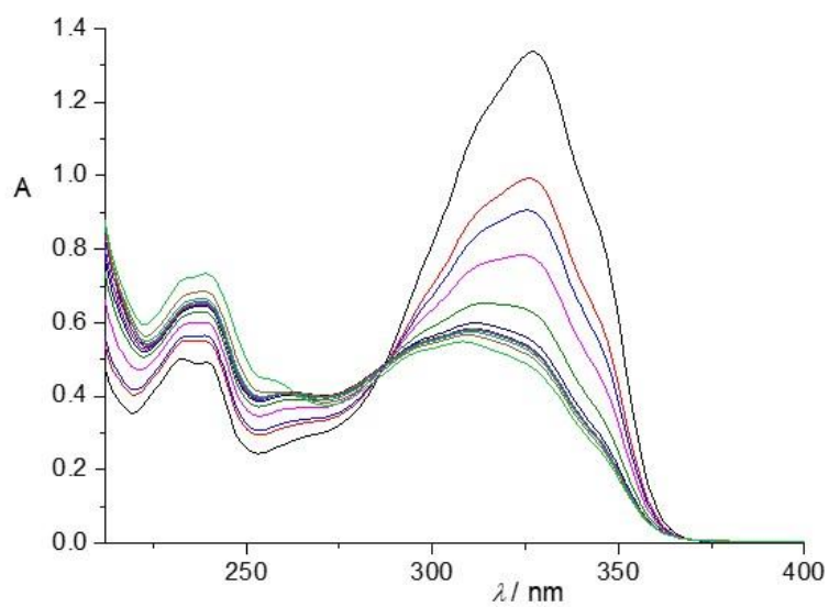
Slika 4. Fotoliza ( E )-2-(4-klorstiril)tiofena ( trans - 1 ) u vremenu 0 – 4096 s (spektar crne boje je početni).
