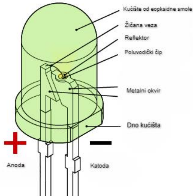
Slika 2. Sastavni dijelovi LED modula 29
