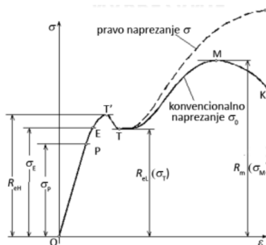
Slika 2.5. Grafički prikaz ovisnosti napreznja ( \sigma ) o istežanju ( \epsilon ) 18
