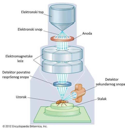
Slika 13. Shematski prikaz SEM-a [23]
