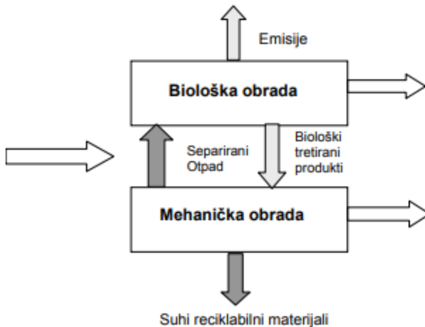
Slika 7. Mehaničko-biološki procesi obzirom na redosljed obrade [13].
