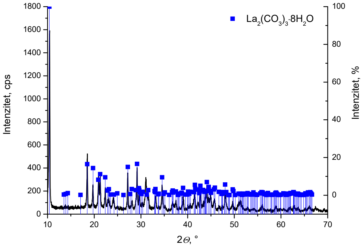
Slika 7. Rezultat rendgenske difrakcijske analize uzorka LSMO_precursor
