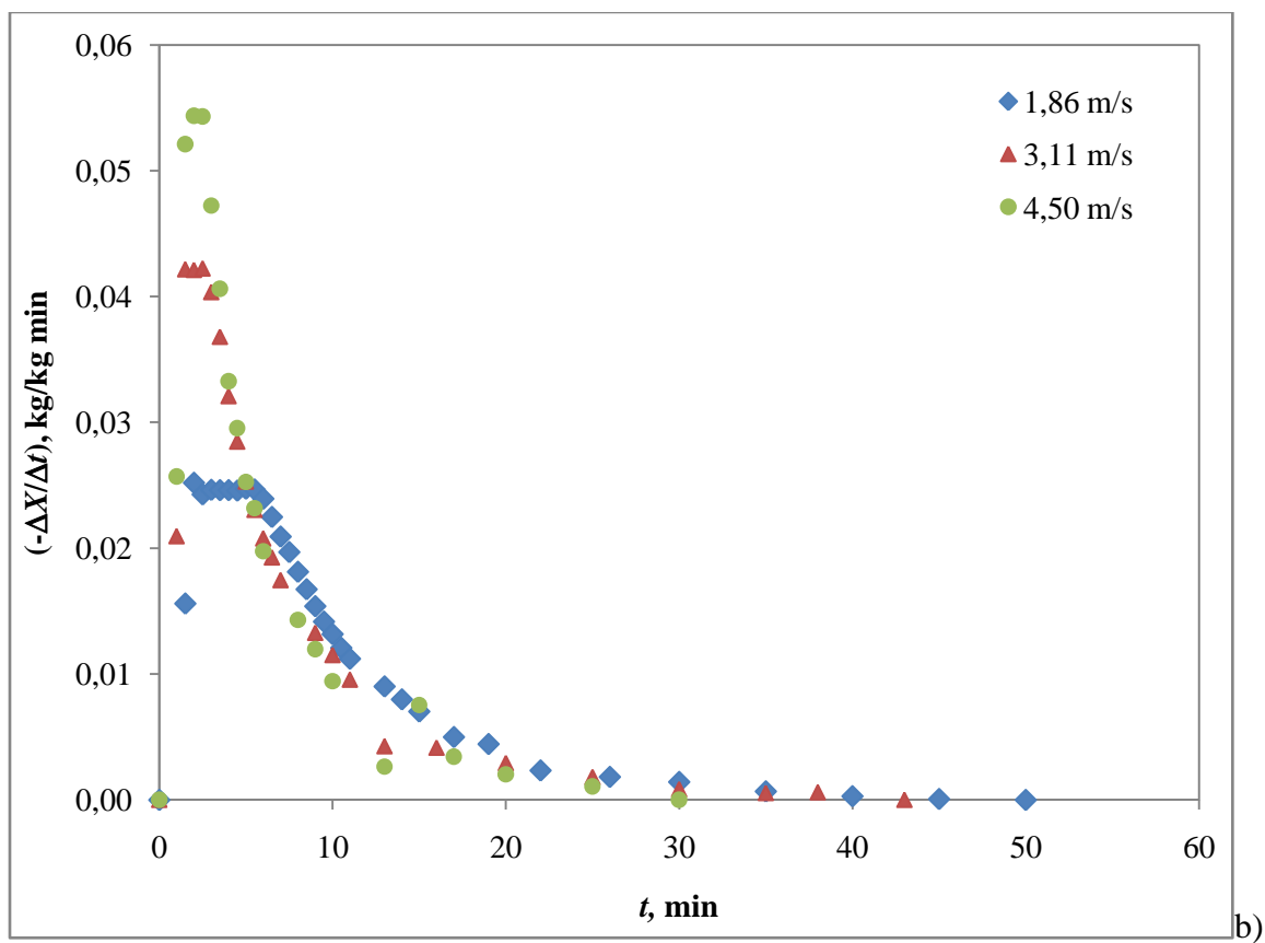
Slika 30. Utjecaj brzine strujanja zraka na kinetiku sušenja (uzorak 3; d=4,05 mm; T=57 °C; (H/D)=1,46 )
