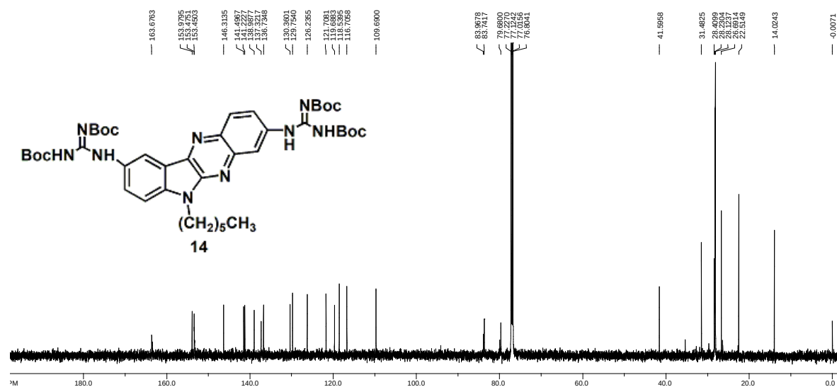
Slika 50. ^{13}\text{C} NMR spektar (CDCl 3 ) spoja 14
