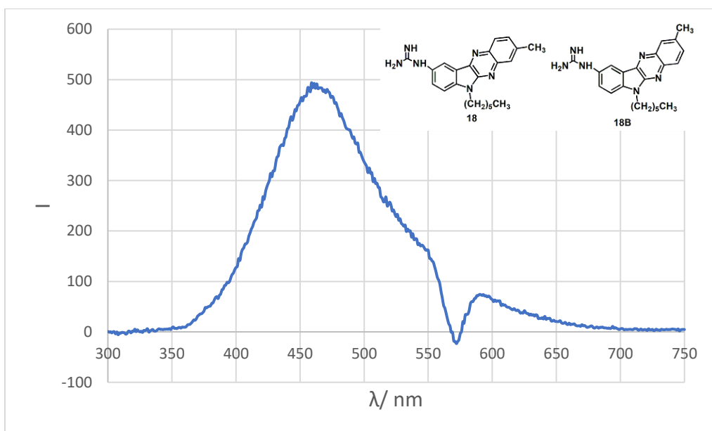
Slika 83. Emisijski spektar ( \text{CH}_3\text{CN} ) smjese 18 i 18B
