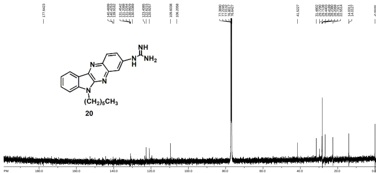
Slika 91. 13 C NMR spektar (CDCl 3 ) spoja 20
