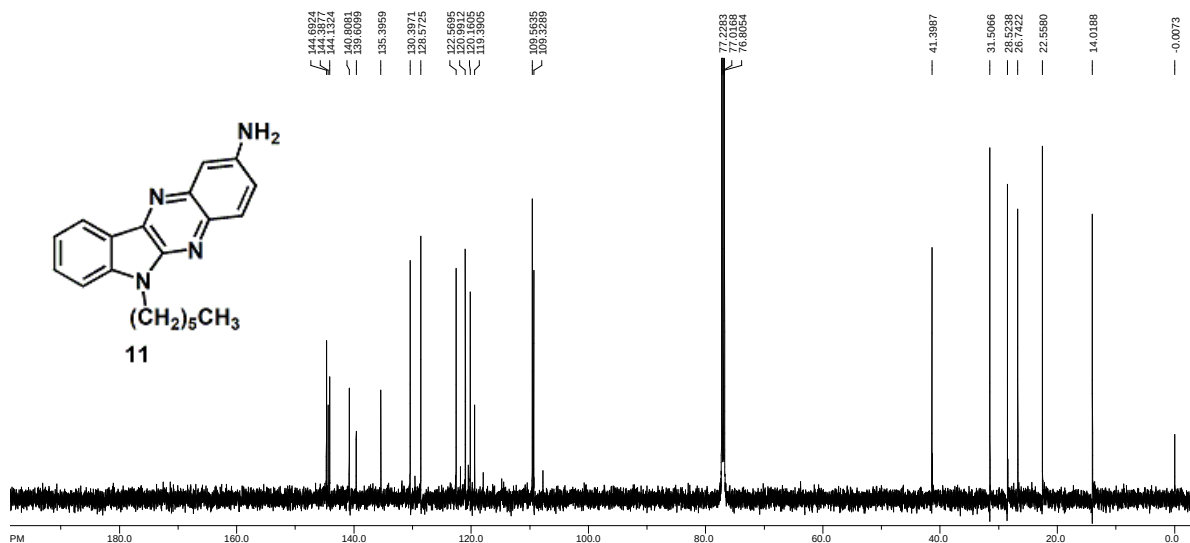
Slika 67. ^{13}\text{C} NMR spektar (CDCl 3 ) spoja 11
