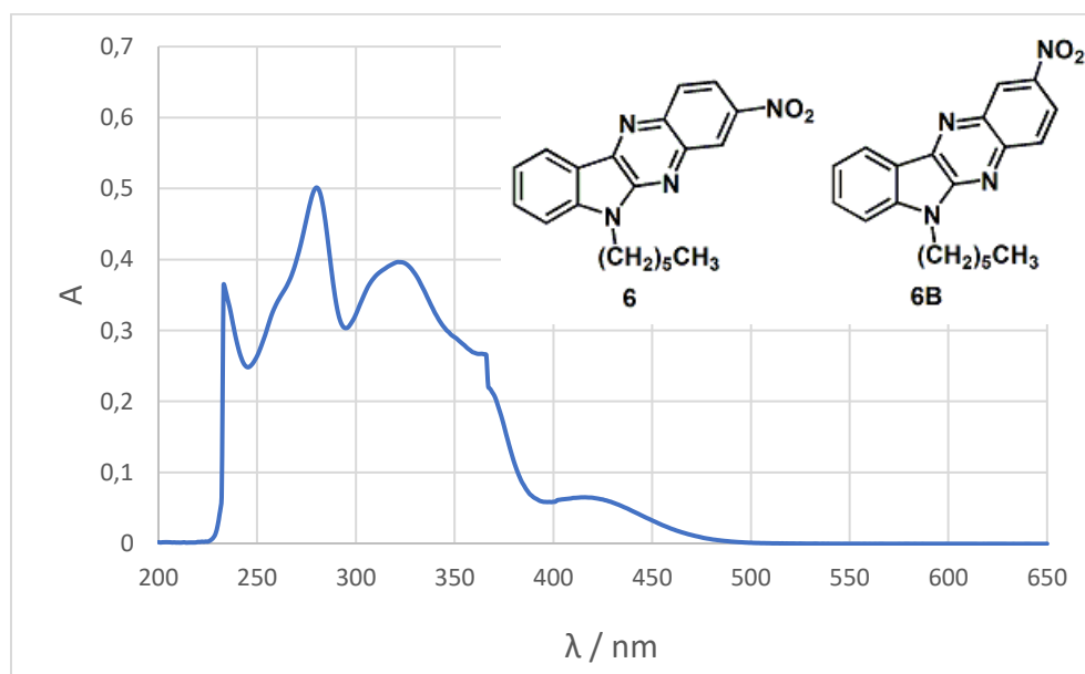
Slika 58. Apsorpcijski spektar (CH 3 CN) smjese 6 i 6B
