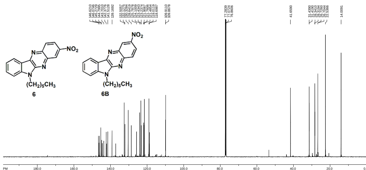
Slika 57. ^{13}\text{C} NMR spektar (CDCl 3 ) smjese 6 i 6B
