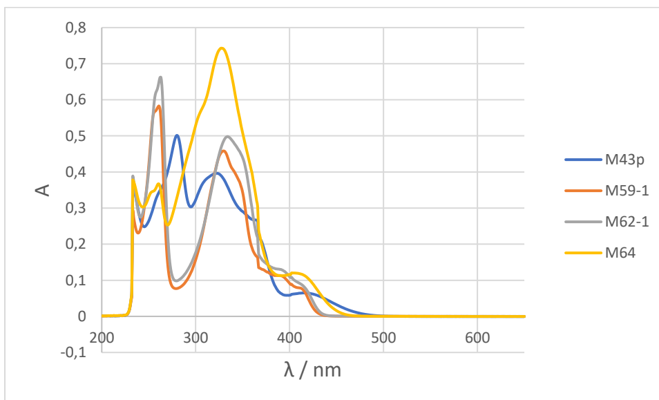
SLIKA 17: Usporedba apsorpcijskih spektara nitro-spojeva
