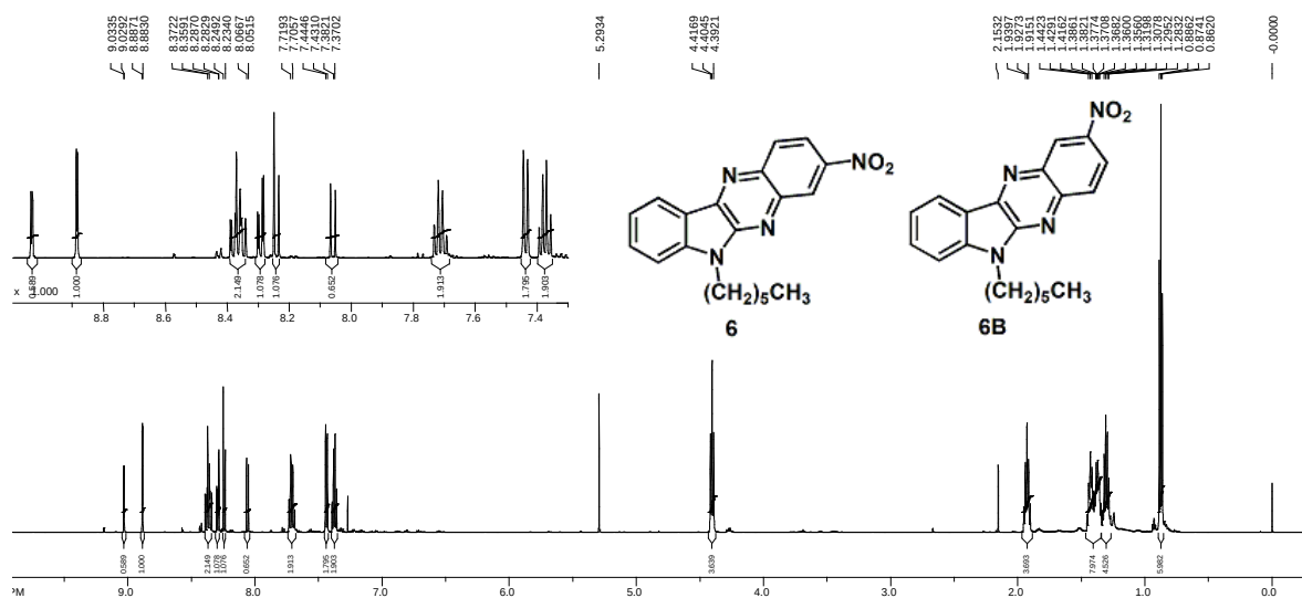
Slika 56. 1 H NMR spektar (CDCl 3 ) smjese 6 i 6B
