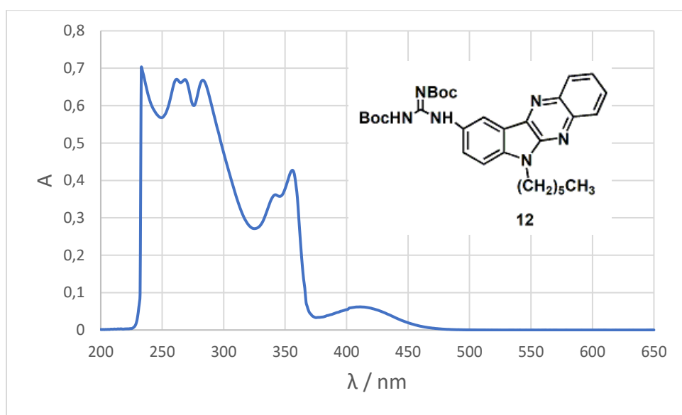
Slika 16. Apsorpcijski spektar (CH 3 CN) spoja 12
