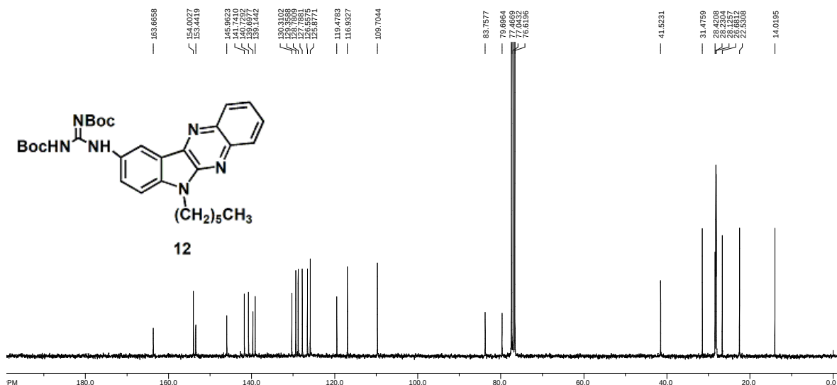
Slika 15. 13 C NMR spektar (CDCl 3 ) spoja 12
