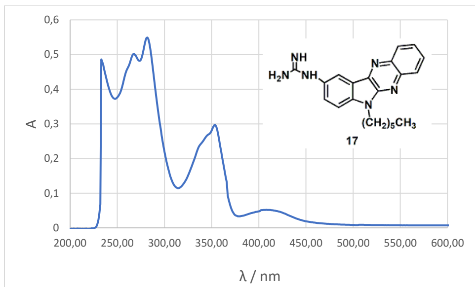
Slika 21. Apsorpcijski spektar (CH 3 CN) spoja 17
