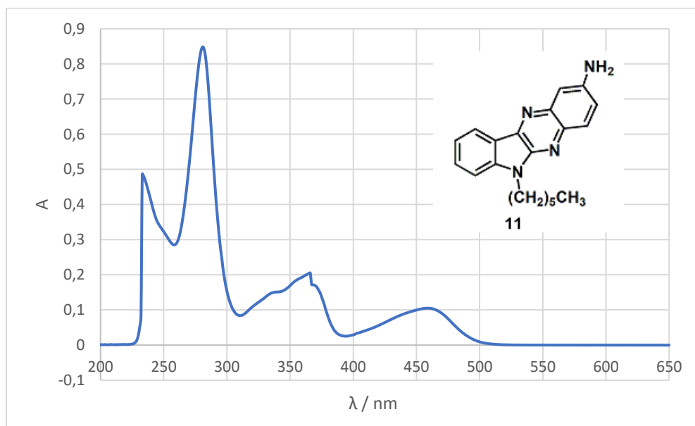
Slika 68. Apsorpcijski spektar (CH 3 CN) spoja 11
