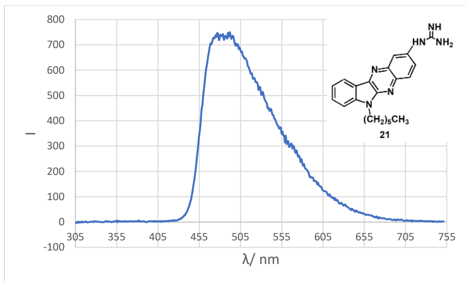
Slika 100. Fluorescencijski spektar ( \text{CH}_3\text{CN} ) spoja 21
