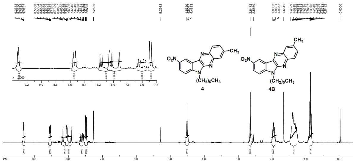
Slika 24. ^1\text{H} NMR spektar ( \text{CDCl}_3 ) smjese 4 i 4B
