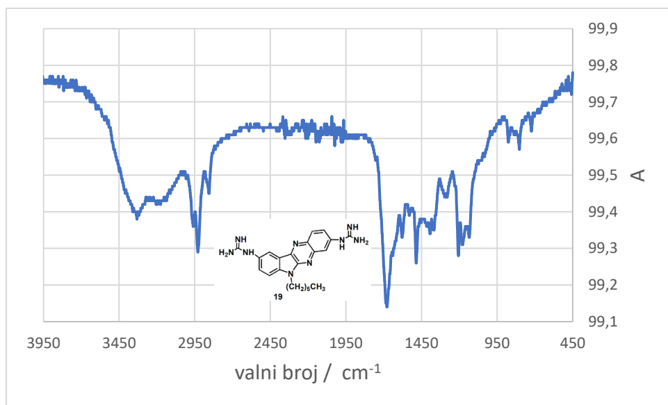
Slika 89. FTIR-ATR spektar spoja 19
