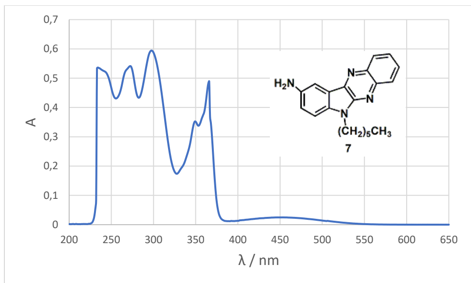
Slika 11. Apsorpcijski spektar ( \text{CH}_3\text{CN} ) spoja 7
