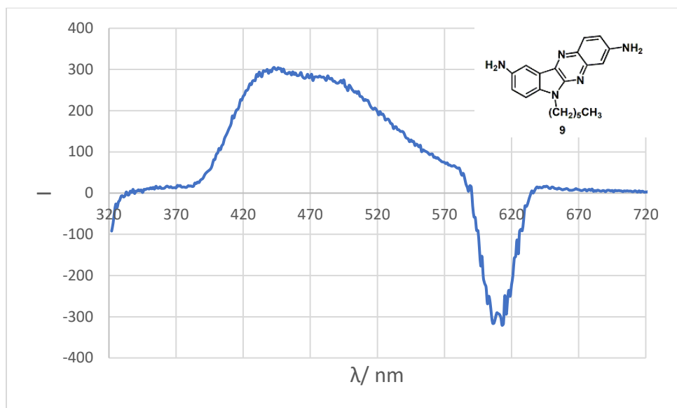
Slika 47. Emisijni spektar ( \text{CH}_3\text{CN} ) spoja 9
