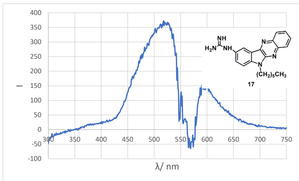
Slika 22. Emisijski spektar (CH 3 CN) spoja 17
