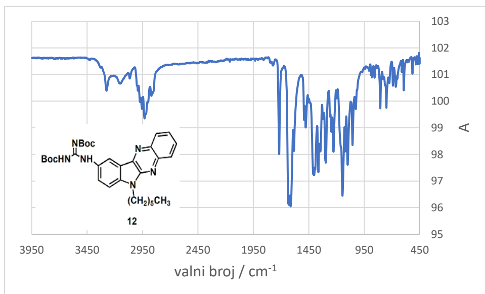
Slika 18. FTIR-ATR spektar spoja 12
