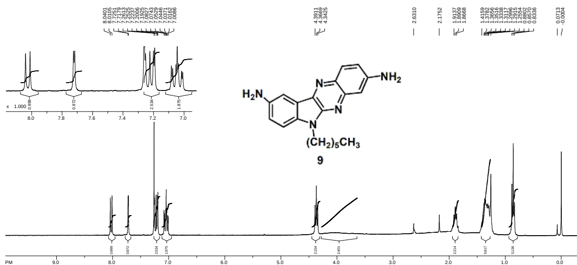
Slika 44. ^1\text{H} NMR spektar ( \text{CDCl}_3 ) spoja 9
