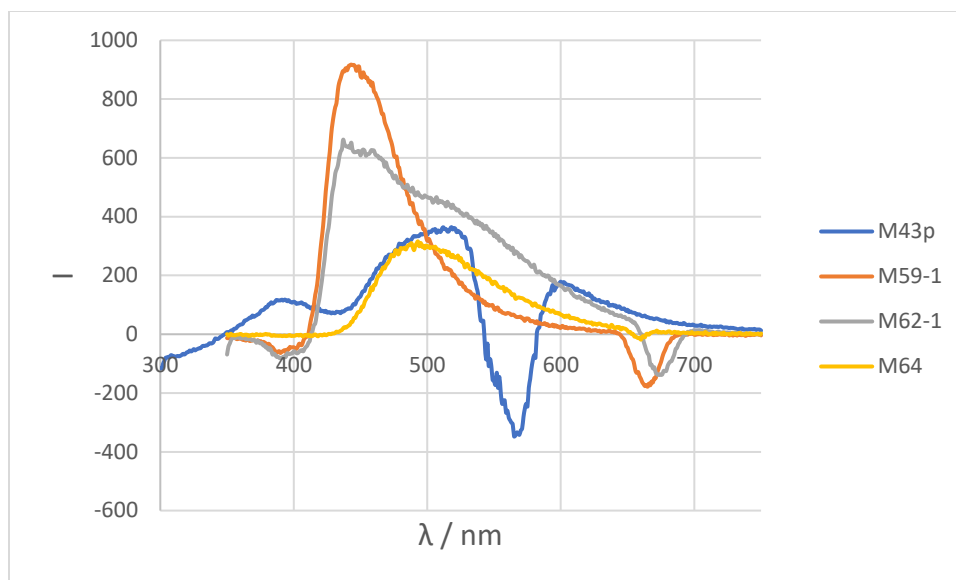
SLIKA 26: Usporedba emisijskih spektara nitro-spojeva
