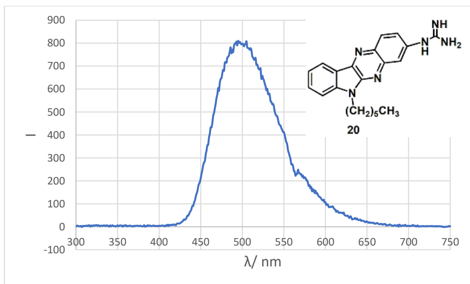
Slika 93. Emisijski spektar (CH 3 CN) spoja 20
