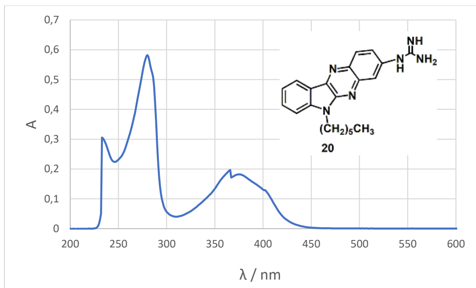
Slika 92. Apsopcijski spektar (CH 3 CN) spoja 20
