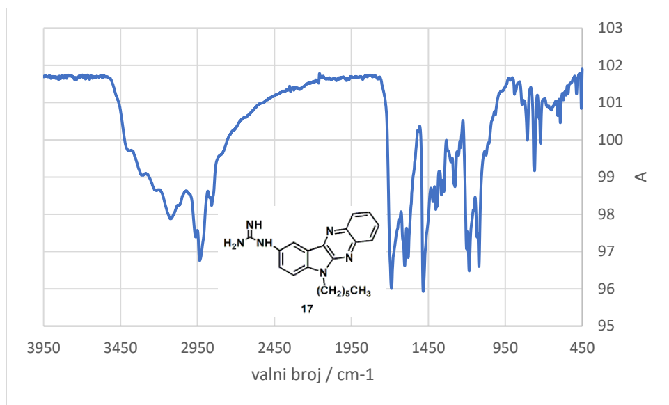
Slika 23. FTIR-ATR spektar spoja 17
