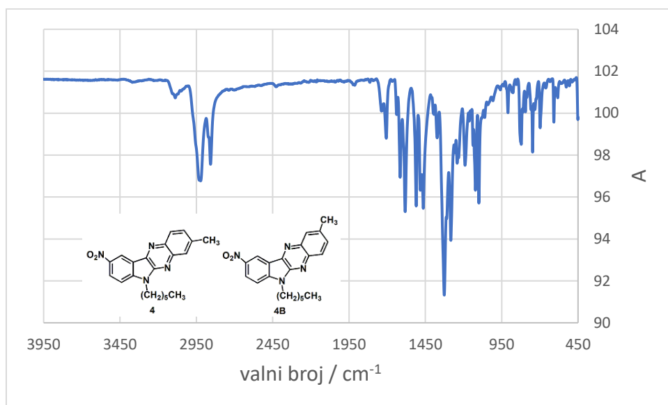
Slika 28. FTIR-ATR spektar smjese 4 i 4B
