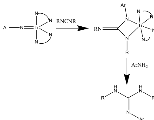
SHEMA 1: Katalitički način sinteze gvanidina (9)
