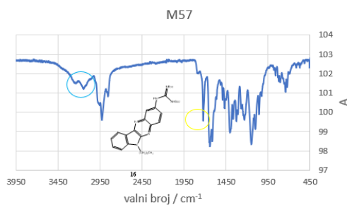
SLIKA 13: IR spektri zaštićenih gvanidina
