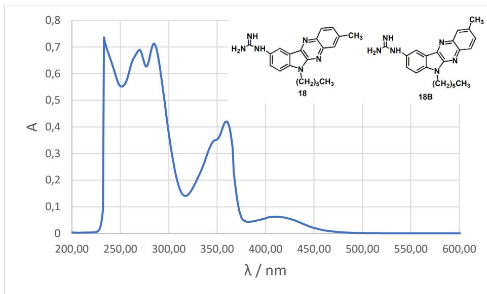
Slika 82. Apsorpcijski spektar ( \text{CH}_3\text{CN} ) smjese 18 i 18B
