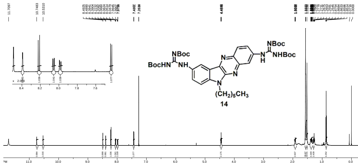
Slika 49. ^1\text{H} NMR spektar (CDCl 3 ) spoja 14
