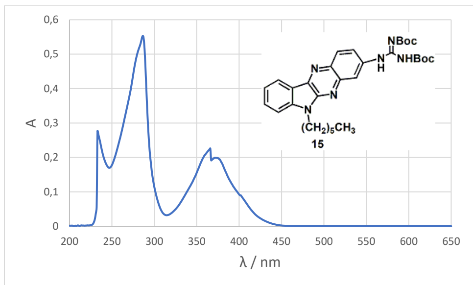
Slika 73. Apsopcijski spektar ( \text{CH}_3\text{CN} ) spoja 15
