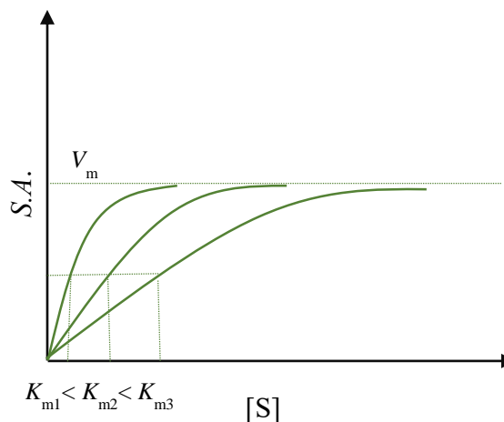
Slika 2. Grafički prikaz MM krivulje za različite vrijednosti K_m
