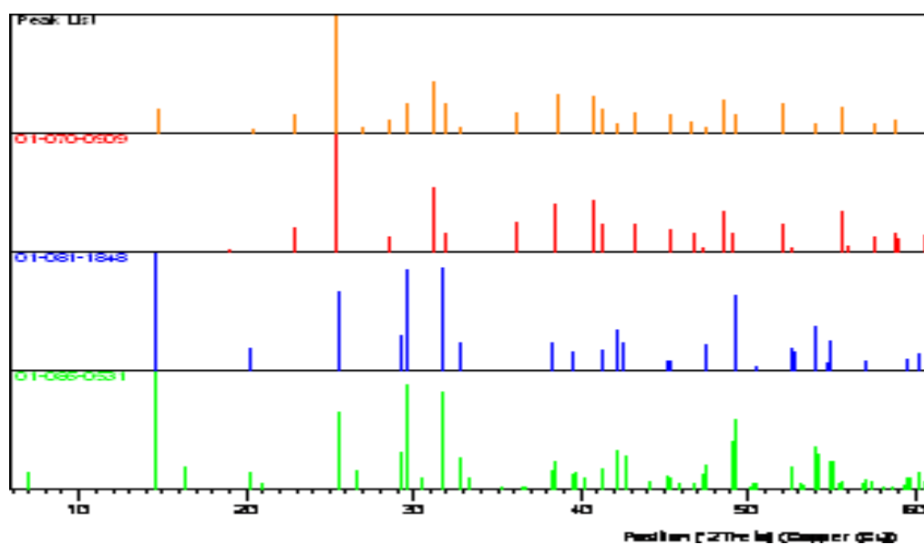
Slika 4.6. Rezultati obrade rezultata rendgenske difrakcijske analize – otpadni gips, 150 °C (otvoren sustav)
