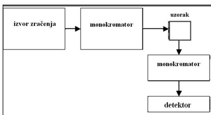
Slika 11. Shema fluorimetra
