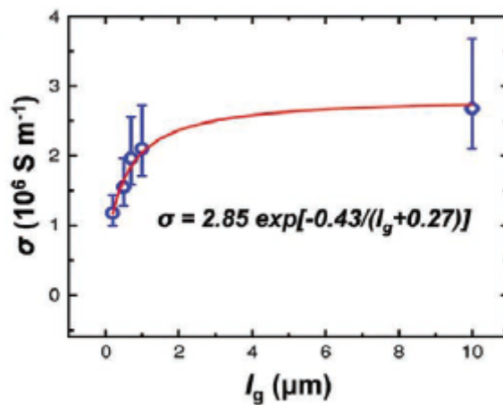
Slika 61. Ovisnost električne vodljivosti grafena o njegovoj veličini 17 .
