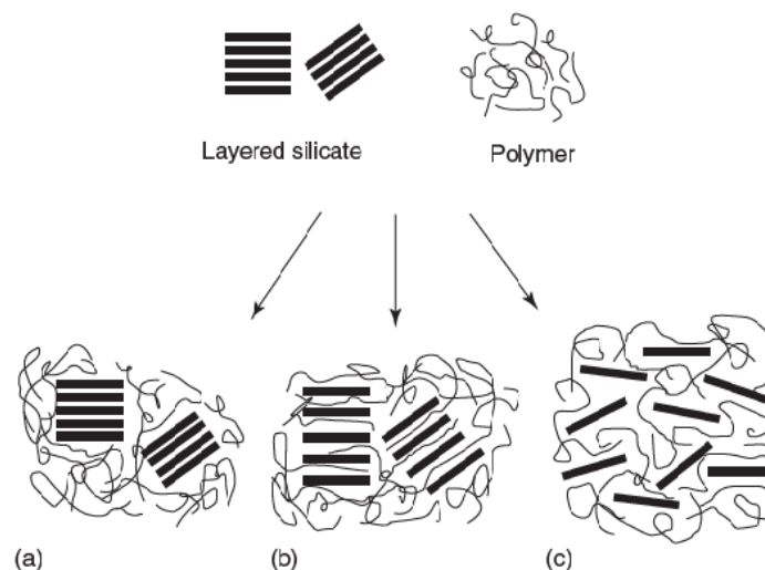
Slika 35. Vrste polimernih mikrostruktura. (a) neinterkalirana (mikrokompoziti). (b) Interkalirana (nanokompoziti). (c) eksfolirana (nanokompoziti) 15 .
