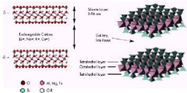
Slika 9. Struktura montmorilonita
