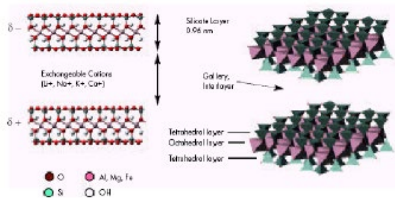
Slika 9. Struktura montmorilonita
