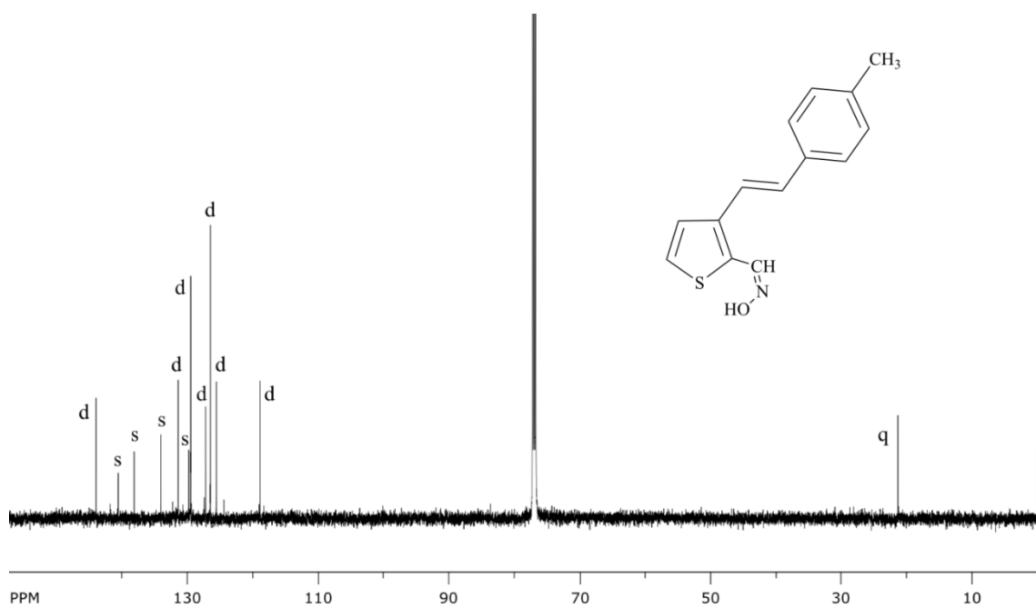
Slika 20. 13 C NMR spektar (Z)-3-((E)-4-metilstil)tiofen-2-karbaldehid oksima ( trans,syn-7 ).
