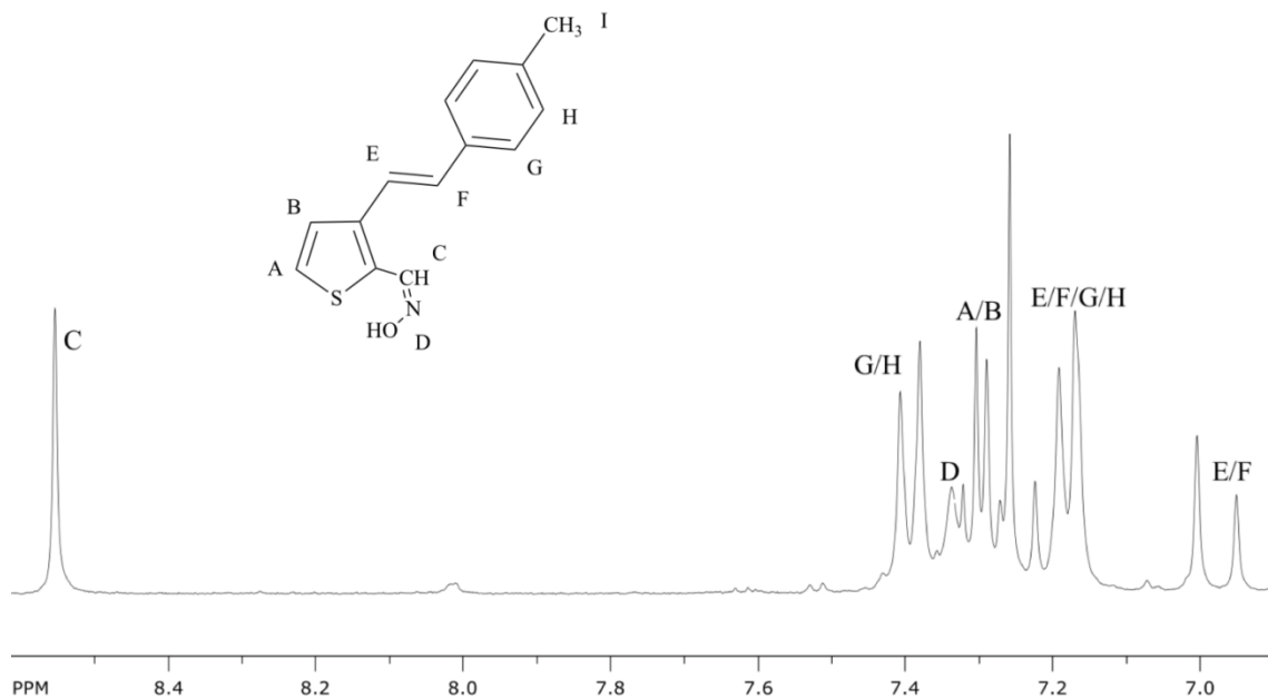
Slika 19. 1 H NMR spektar (Z)-3-((E)-4-metilstil)tiofen-2-karbaldehid oksima ( trans,syn-7 ).
