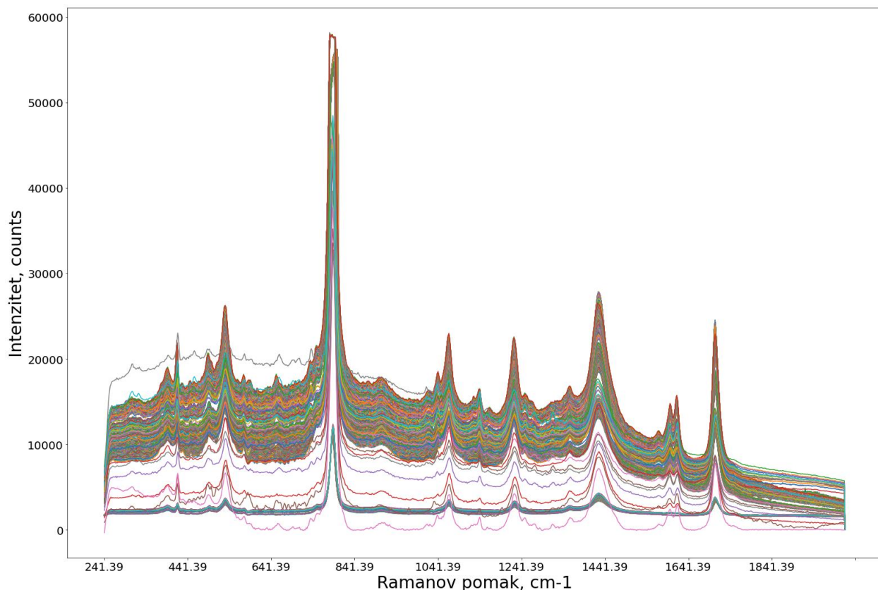
Slika 32. Ramanovi spektri
