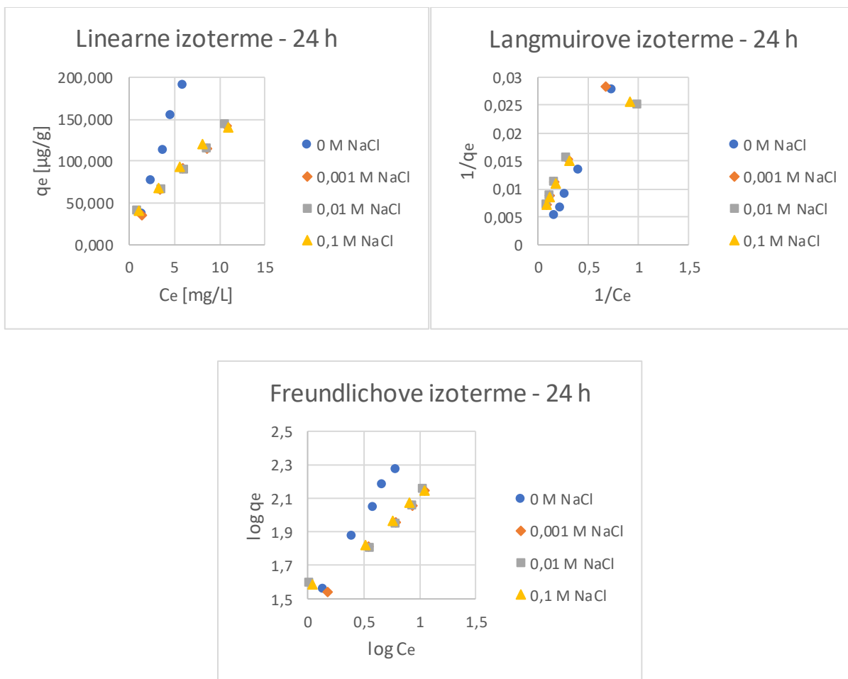
Slika 27. Imatinib: Grafički prikazi sorpcijskih izoterme nakon 24 sata mućkanja za različite ionske jakosti ( c(\text{NaCl}) = 0 \text{ M}, 0,001 \text{ M}, 0,01 \text{ M}, 0,1 \text{ M} )
