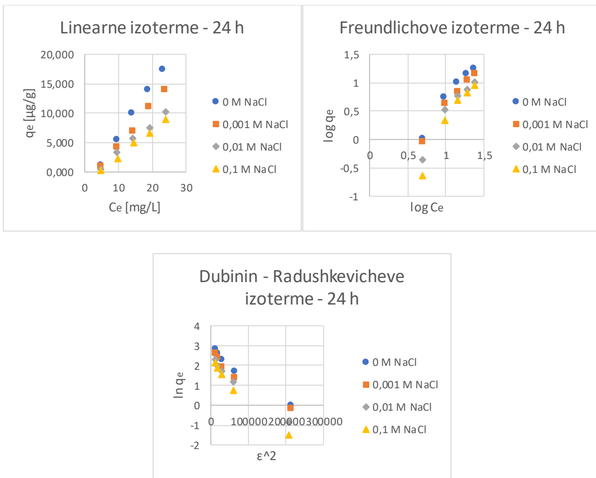
Slika 28. Torasemid: Grafički prikazi sorpcijskih izotermi nakon 24 sata mućkanja za različite ionske jakosti ( c(\text{NaCl}) = 0 \text{ M}, 0,001 \text{ M}, 0,01 \text{ M}, 0,1 \text{ M} )
