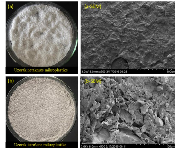
Slika 18. Fotomikrografske slike čestica netaknute i ostarjele polistirenske pjene i njihove mikroskopske površinske morfologije [17].
