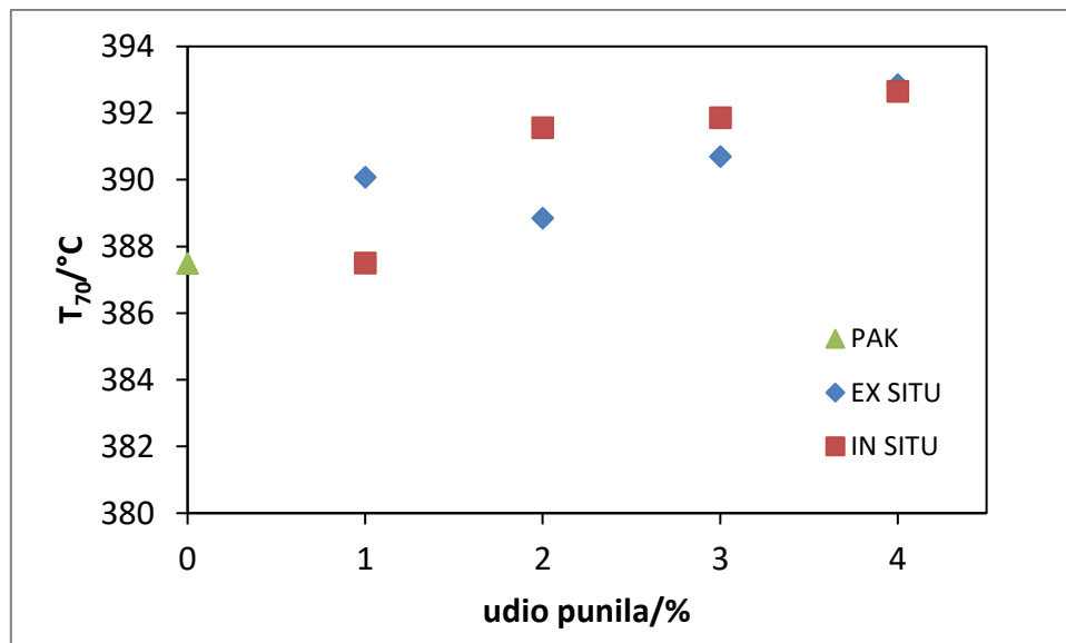
Slika 40. Temperature pri kojima gubitak mase iznosi 30 %
