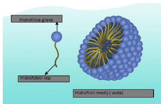
Slika 2. Micela emulgatora [12]
