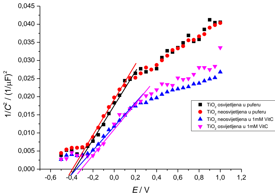
Slika 4.9 Grafički prikaz Mott-Schottky analize za osvijetljenu i neosvijetljenu TiO_2 elektrodu u puferu i vitaminu C koncentracije 1 \text{ mmol dm}^{-3} pri frekvenciji od 1 kHz.
