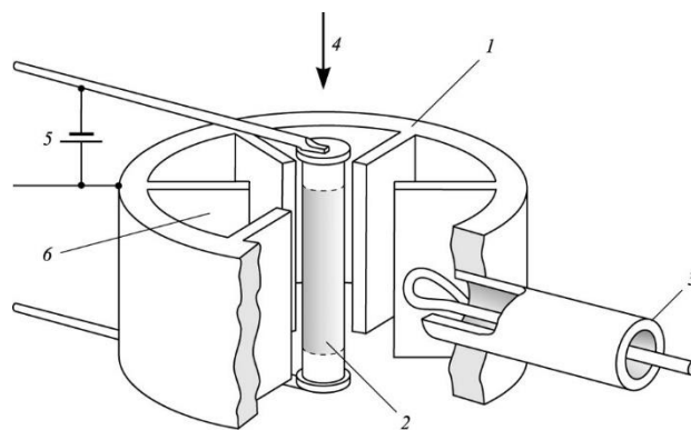
Slika 7. Dijelovi magnetrona: 1. anoda, 2. katoda, 3. koaksijalna linija na izlazu, 4. smjer magnetskoga polja, 5. anodni napon, 6. rezonantna šupljina [87]
