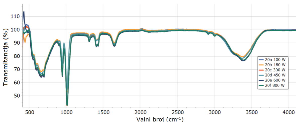
Slika 49. FTIR spekter uzorka 20 nakon pripadajućeg mikrovalnog zračenja (20A- 100 W, 20B- 180 W, 20C- 300 W, 20D- 450 W, 20E- 600 W i 20F- 800 W)
