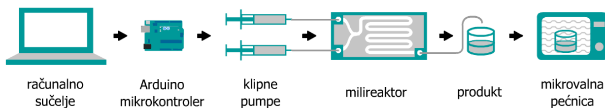
Slika 16. Shematski prikaz procesa sinteze pomoću milireaktora potpomognute mikrovalnim zračenjem.
