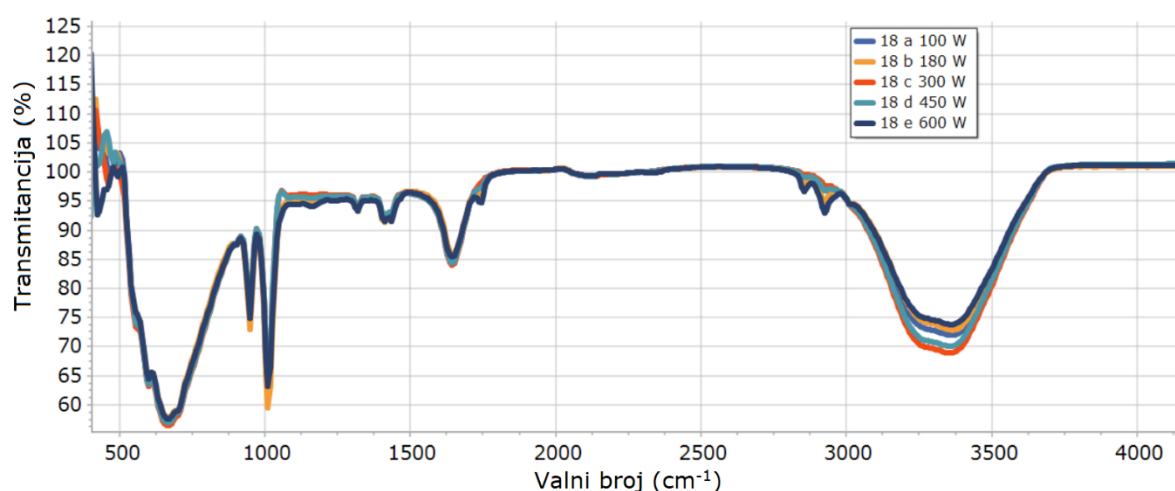
Slika 44. Uzorak 18 nakon raspodjele u 6 bočica i pripadajućeg mikrovalnog zračenja (18A- 100 W, 18B- 180 W, 18C- 300 W, 18D- 450 W, 18E- 600 W i 18F- 800 W)
