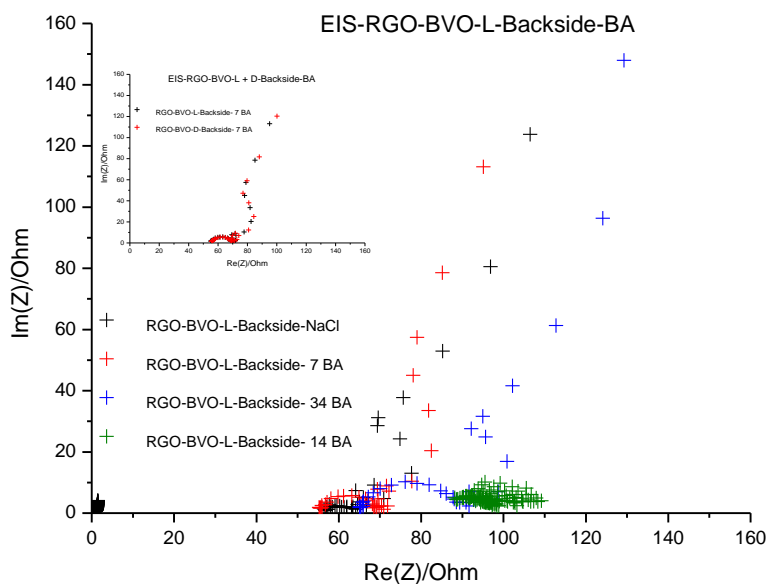
Slika 42. Nyquistov prikaz ovisnosti imaginarni komponente o realnoj komponenti impedancije za rGO-BVO elektrodu u 0,1 \text{ M} otopini NaCl i otopinama benzojeve kiseline masenih koncentracija 7 \text{ mgL}^{-1} , 14 \text{ mgL}^{-1} i 34 \text{ mgL}^{-1} . Na manjem grafu dan je Nyquistov prikaz za osvjetljenu i neosvjetljenu rGO-BVO elektrodu u otopini benzojeve kiseline masene koncentracije 7 \text{ mgL}^{-1} .
