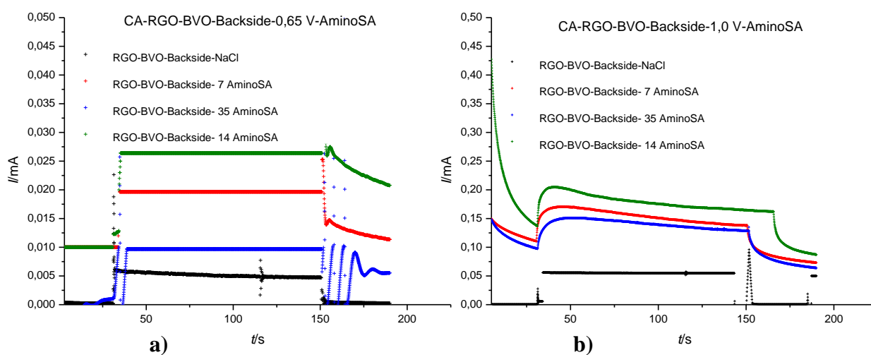
Slika 59. Grafički prikaz ovisnosti struje o vremenu za rGO-BVO elektrodu u 0,1 M otopini NaCl i otopinama aminosalicilne kiseline masenih koncentracija 7 mgL -1 , 14 mgL -1 i 35 mgL -1 pri potencijalima od a) 0,65 V i b) 1,0 V.
