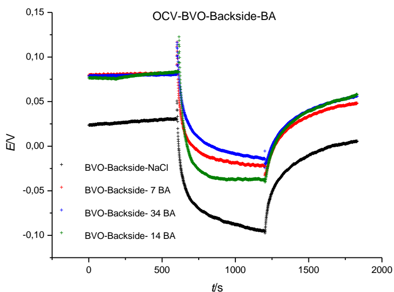
Slika 62. Grafički prikaz promijene potencijala otvorenog kruga s vremenom za BVO elektrodu u u 0,1 M otopini NaCl i otopinama benzojeve kiseline masenih koncentracija 7 mgL -1 , 14 mgL -1 i 34 mgL -1 .
