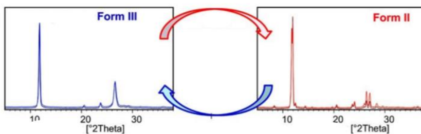
Slika 6. Utjecaj polimorfije na difrakcijsku sliku. 20
