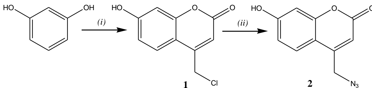
Shema 1. (i) etil-4-kloroacetoacetat, \text{H}_2\text{SO}_4 (konc.), (ii) \text{NaN}_3 , \text{CH}_3\text{CN}
