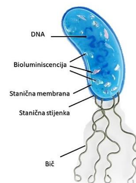
Slika 2.5. Bakterija Vibrio fischeri (preuzeto i prilagođeno) [56]
