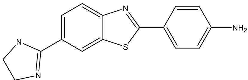
Slika 4.57. Prikaz molekulske strukture razgradnog produkta m/z 293 ( t_R=7,344 min)
