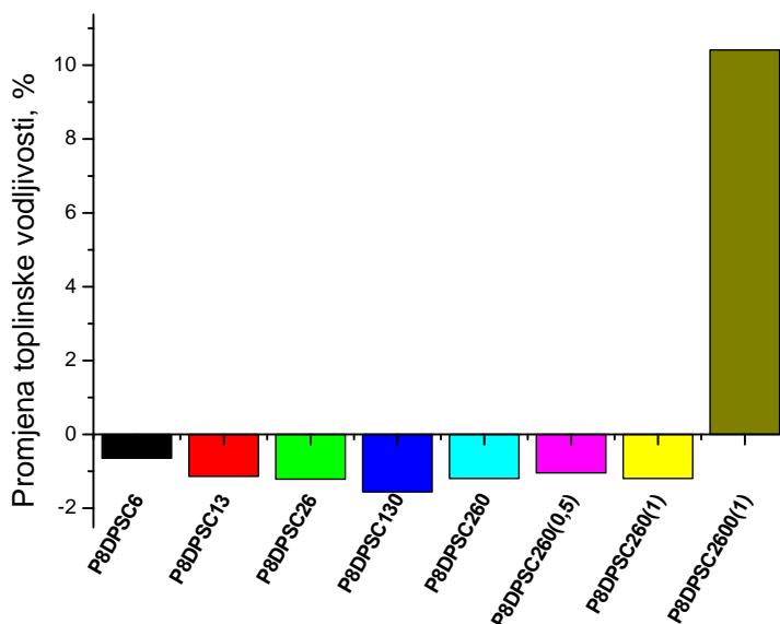
Slika 4.4.1. Postotna promjena toplinske vodljivosti uzoraka u odnosu na PAO 8 ulje
