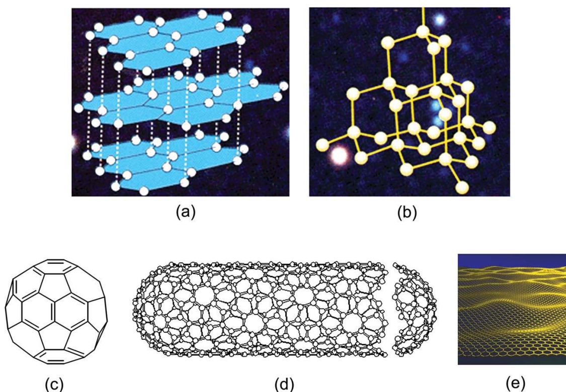
Slika 2.2.1. Alotropske modifikacije ugljika : a) grafit, b) dijamant, c) Buckminster fullerene C_{60} , d) ugljikova nanocijevi i e) grafen
