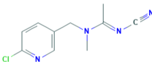
Slika 2.1. Struktura acetamiprida [10]
