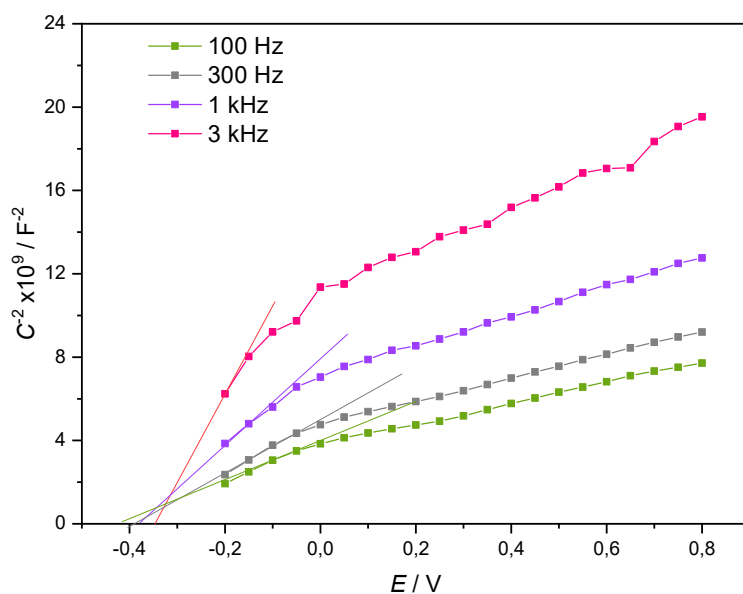
Slika 46. Mott-Schottky prikaz pri različitim frekvencijama. Krivulje su snimljene uz \text{TiO}_2 katalizator u otopini NaCl, raspon potencijala -0,2 – 0,8 V i amplitudu pobude potencijala 5 mV.
