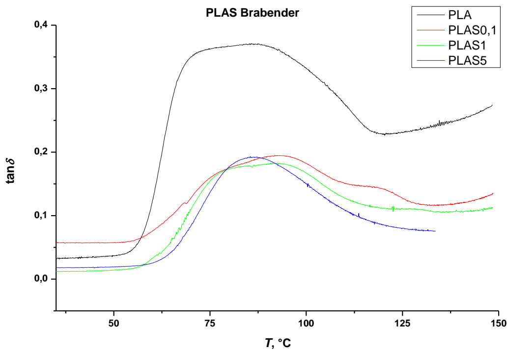
Slika 4.7. Tangens kuta faznog pomaka u ovisnosti o temperaturi za PLA i PLAGL kompozite Brabender serije
