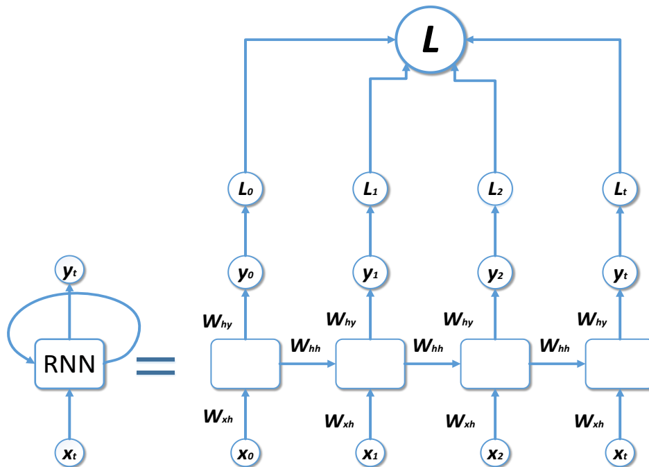
Slika 17. Rekurentna neuronska mreža odmotana u vremenu
