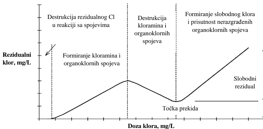
Slika 5. Shematski prikaz tijekom procesa klorinacije
