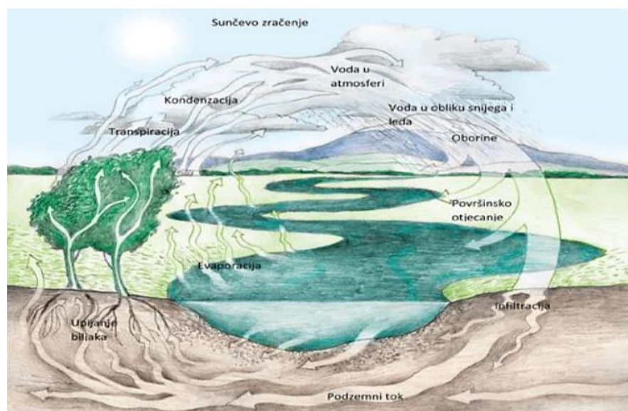
Slika 1. Hidrološki ciklus
