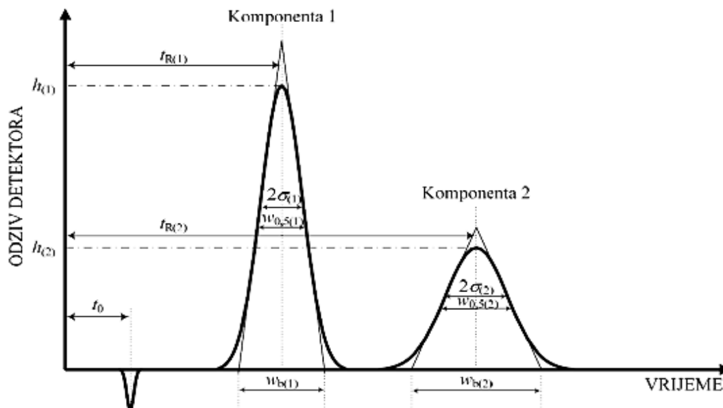
Slika 10. Tipičan prikaz kromatograma
