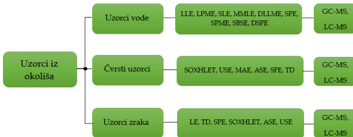
Slika 2. Shematski prikaz uobičajenog postupka analize ftalata iz različitih uzoraka okoliša
