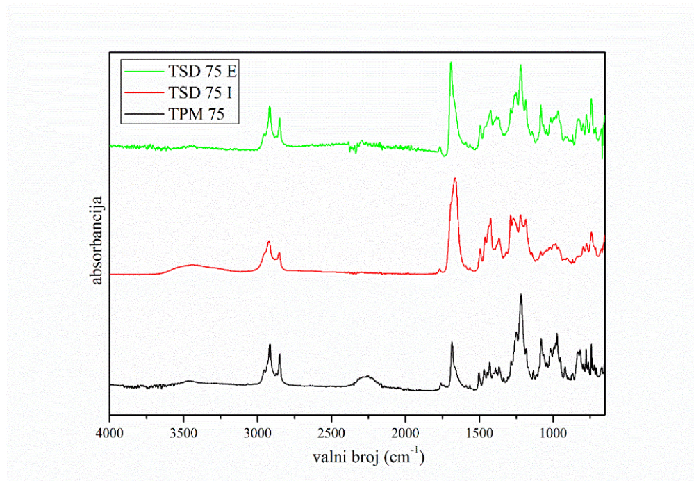
Slika 5.10. FTIR spektri ternarnih fizikalnih mješavina i čvrstih disperzija u kojemu je omjer djelatne tvari naspram polimera 75:25.
