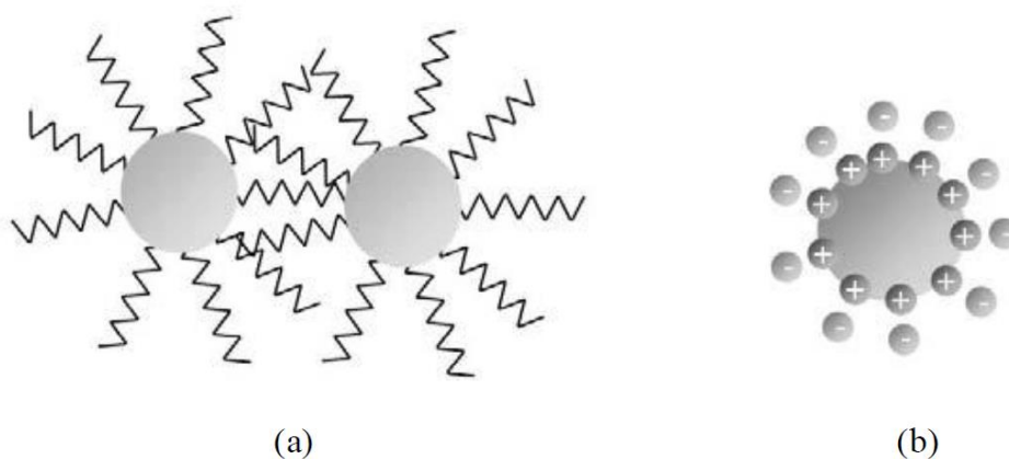
SLIKA 4.: Osnovni načini stabilizacije koloida: (a) sterička; (b) elektrostatska stabilizacija [6].
