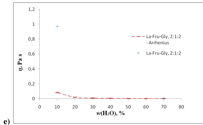
Slika 15. Usporedba Arrheniusovog modela s eksperimentalnim podacima za a) La-Gly, 2:1, b) La-Gly, 1:2, c) La-Gly, 1:1, d) Ma-Gly, 1:4, e) La-Fru-Gly, 2:1:2
