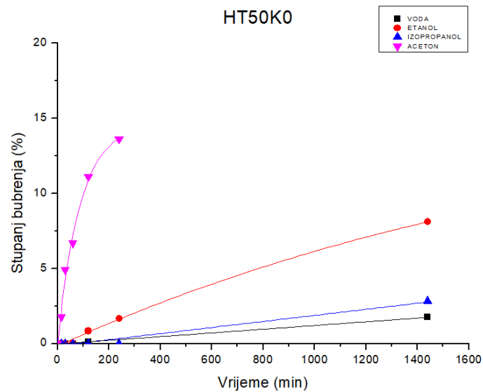
Slika 32. Ovisnosti stupnja bubrenja (u otapalima vodi, etanolu, izopropanolu i acetonu) o vremenu za epruvete od materijala High Temp (HT), debljine ispisa 50 \mu\text{m} , ispisane pod 0° (K0).
