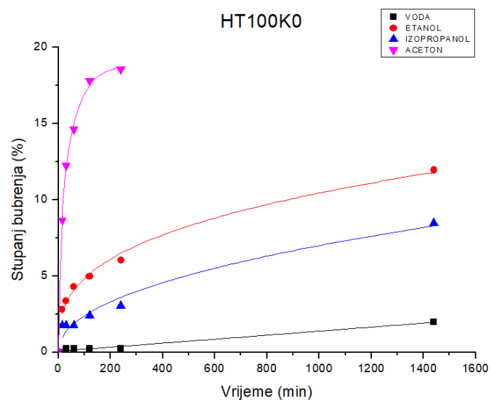
Slika 33. Ovisnosti stupnja bubrenja (u otapalima vodi, etanolu, izopropanolu i acetonu) o vremenu za epruvete od materijala High Temp (HT), debljine ispisa 100 \mu\text{m} , ispisane pod 0° (K0).
