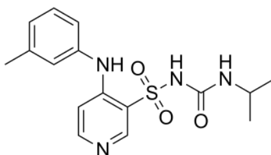
Slika 2.1. Struktura torasemida
