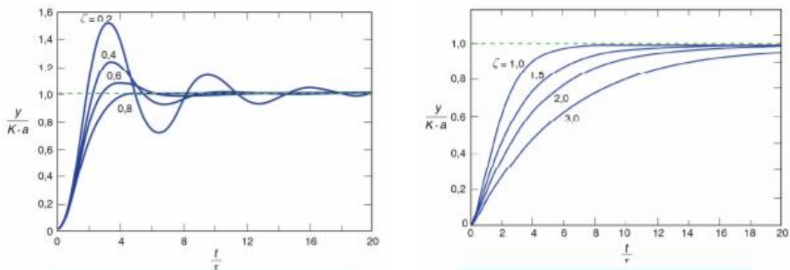
Slika 15 Prikaz neprigušenog i prigušenog odziva procesa drugog reda 11
