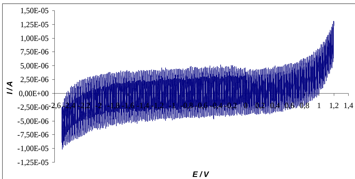
Slika 4.3. Ciklički voltamogram za Al elektrodu u 0,1 M otopini \text{LiPF}_6 u otapalu propilen karbonatu
