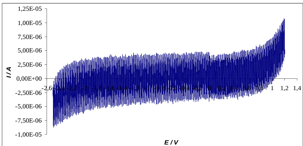
Slika 4.4. Ciklički voltamogram za Al elektrodu u 0,1 M otopini \text{LiPF}_6 u smjesi otapala propilen karbonata i etilen karbonata koji su pomiješani u volumnom omjeru 50:50
