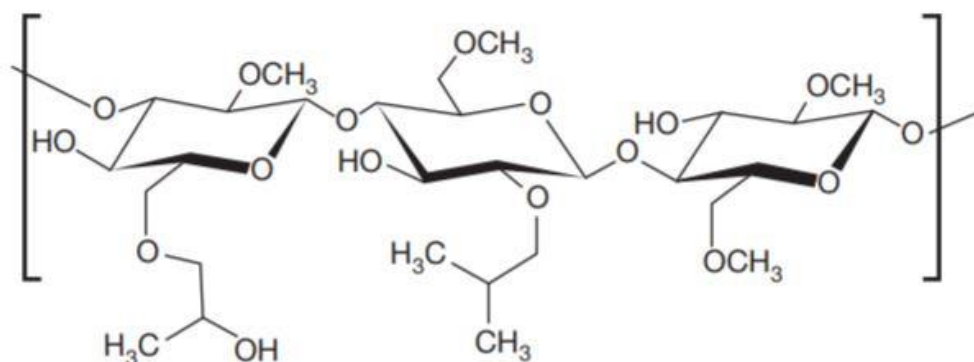
Slika 3.3. Struktura HPMC-a 19
