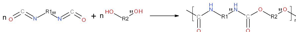
Slika 5. Shematski prikaz nastajanja poliuretana
