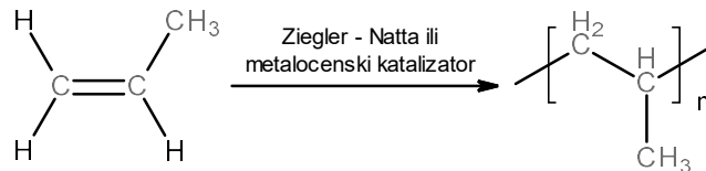
Slika 3. Polimerizacija propena
