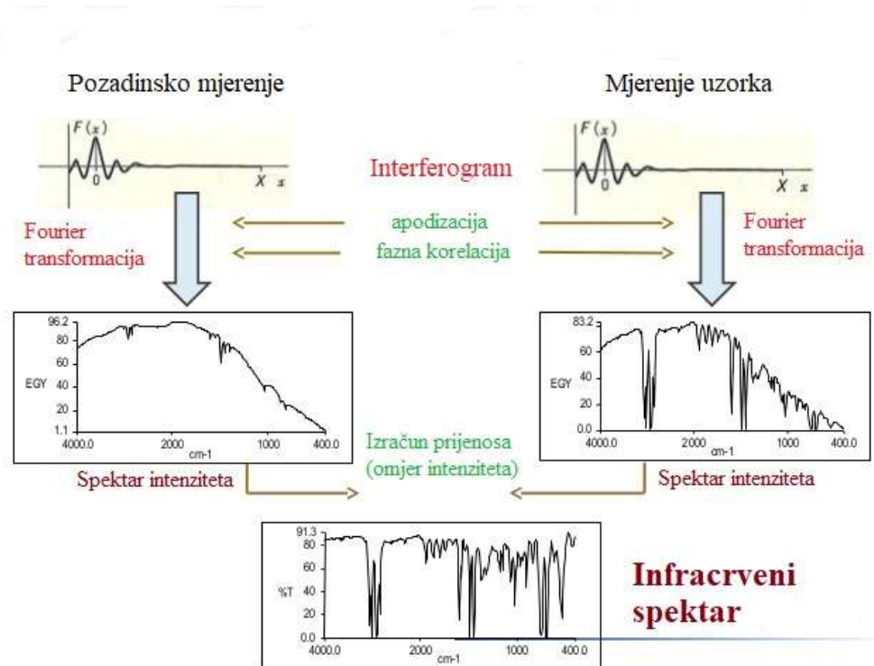
Slika 13. Shematski prikaz Fourierove transformacije
