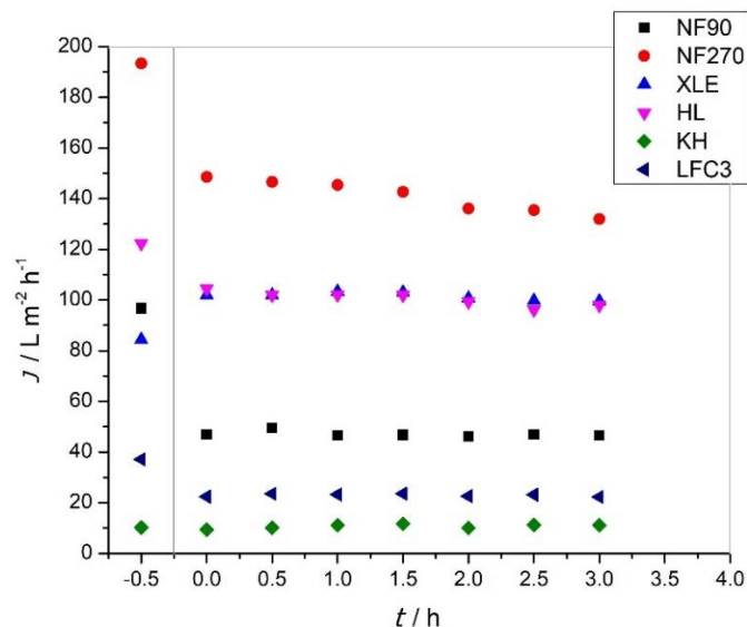
Slika 10. Fluks permeata febantela kroz membrane tijekom 3 h rada
