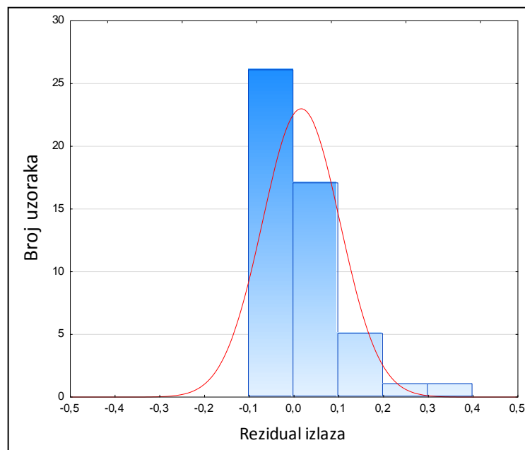
Slika 19 Histogram reziduala izlaza MARSSpline modela (mali skup podataka)
