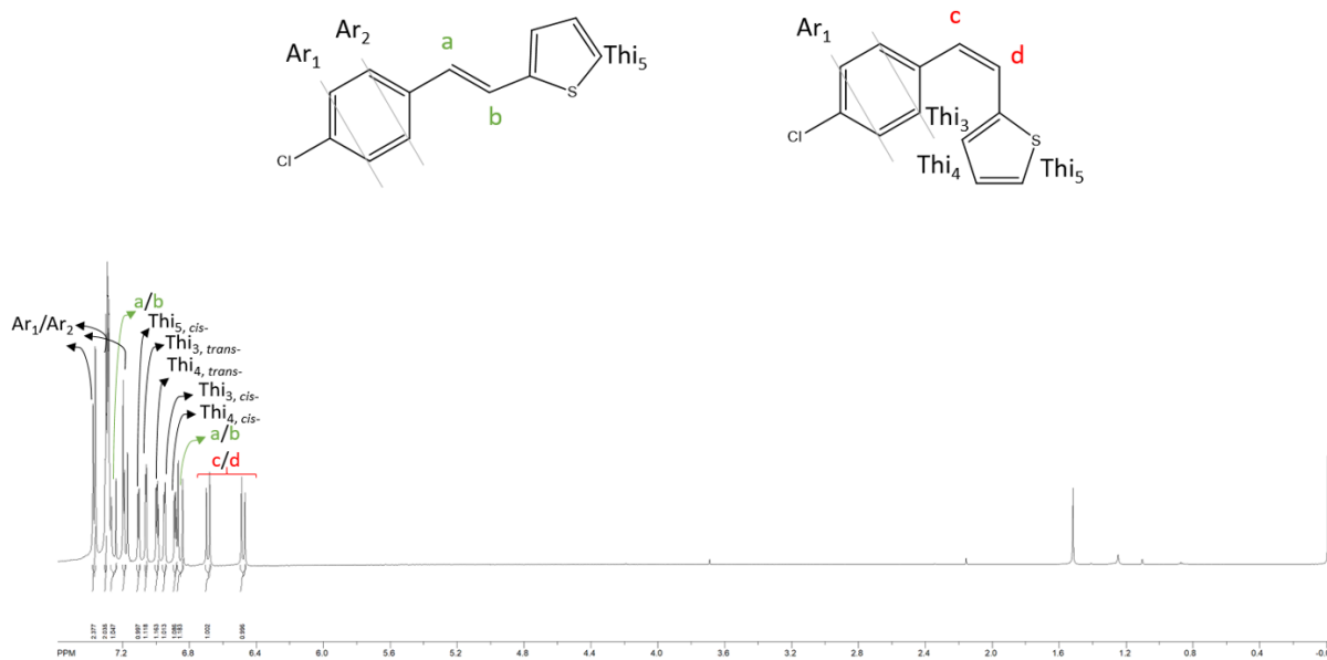
Slika 6. ^1\text{H} NMR spektar 2-(4-klorstiril)tiofena ( 1 ).
