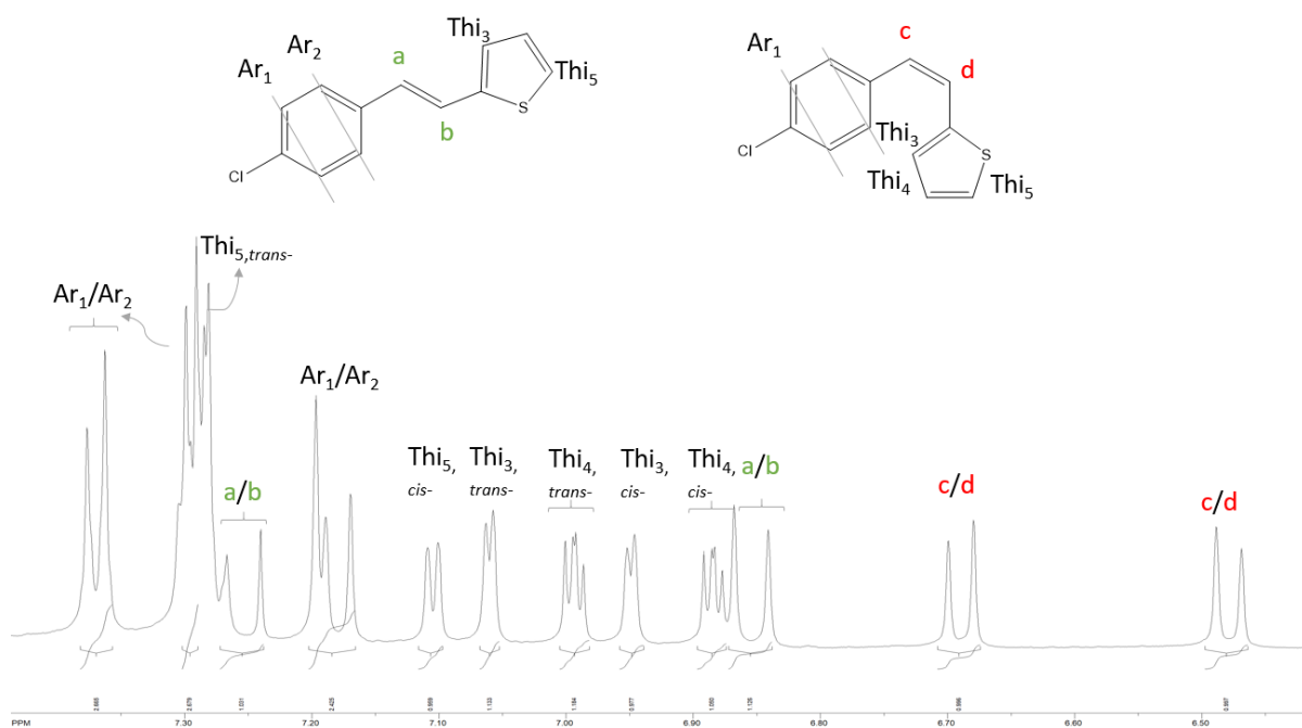
Slika 7. Uvećani prikaz ^1\text{H} NMR spektra 2-(4-klorstiril)tiofena ( 1 ).
