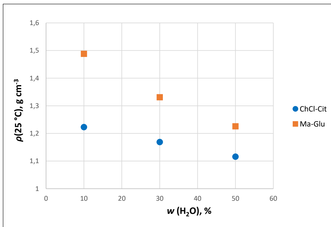
Slika 11. Gustoća u ovisnosti o masenim udjelima vode NADES-a ChCl-Cit i Ma-Glu pri temperaturi od 25 °C.
