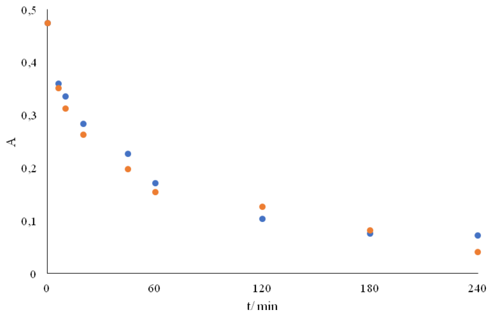
Slika 32. Promjena apsorbancije nitrofurantoina tijekom heterogene fotokatalitičke razgradnje u struji kisika (●) te argona (●) za vrpcu pri 268 nm
