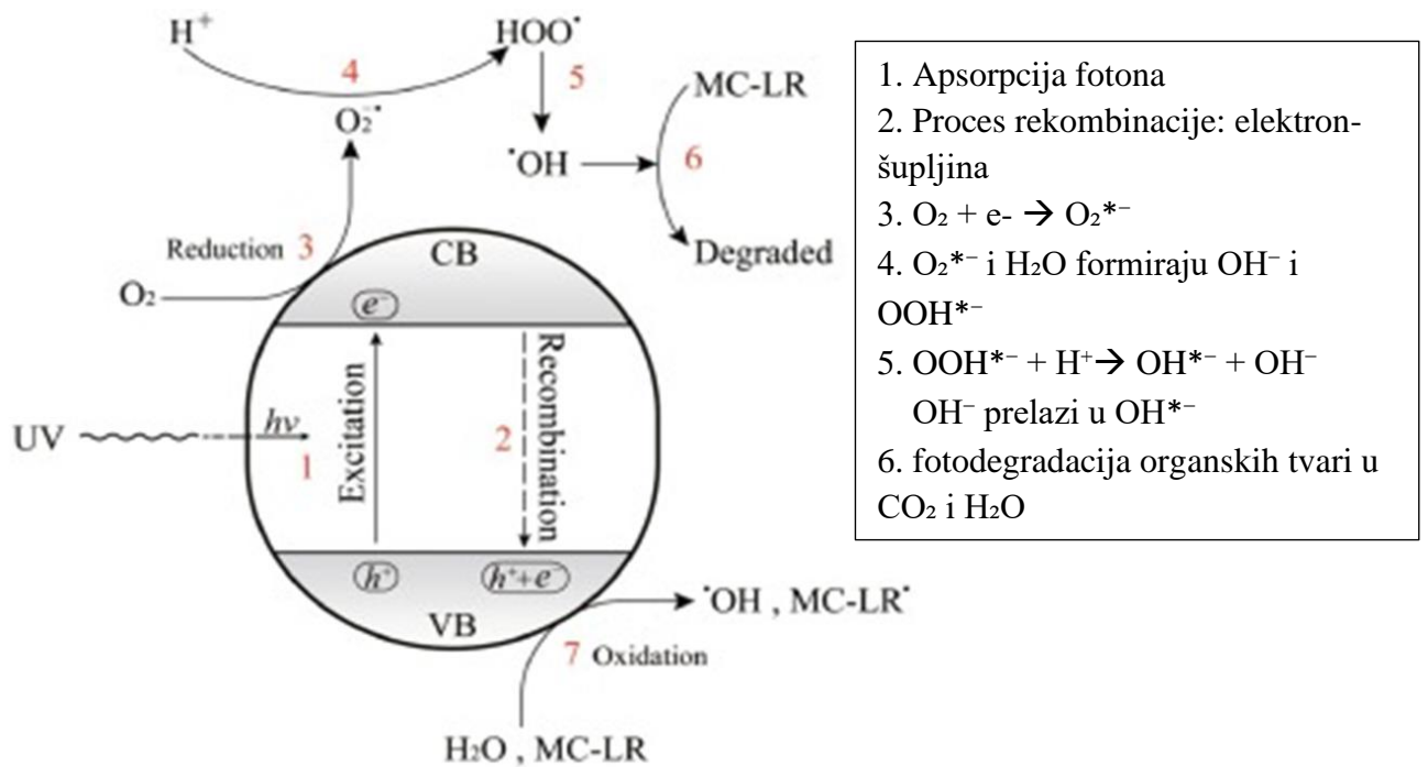
Slika 12. Mehanizam oksidativne razgradnje prilikom pročišćavanja vode [43]
