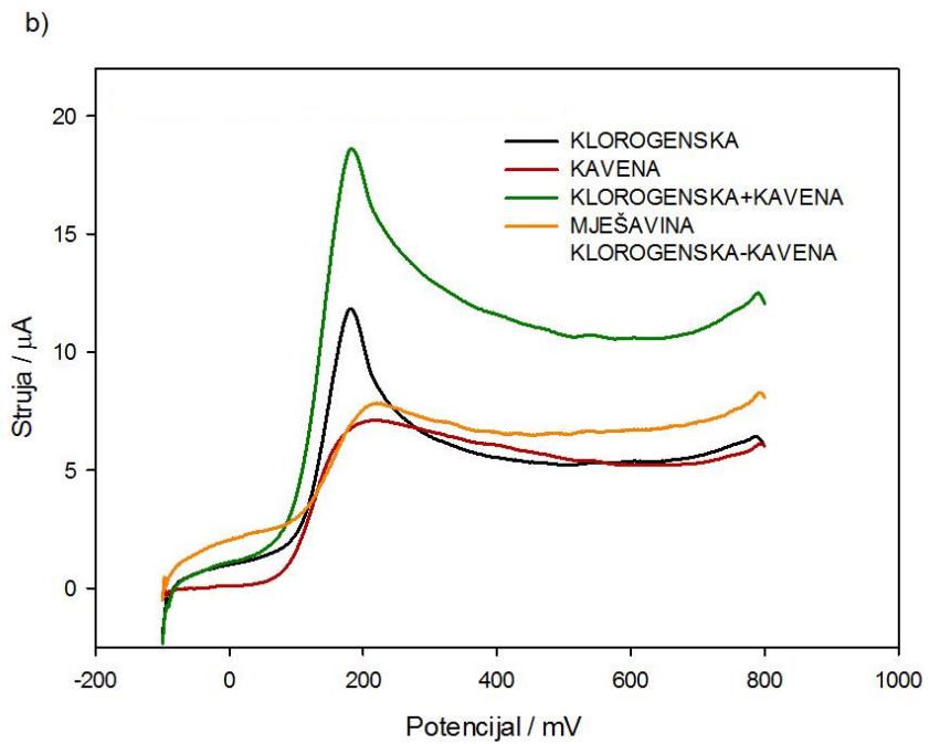
Slika 4.15. Odziv mješavine klorogenske i kavene kiseline u usporedbi sa odzivima pojedinačnih kiselina te zbrojem njihovih signala pod a) sobnim osvjetljenjem i b) UV lampom
